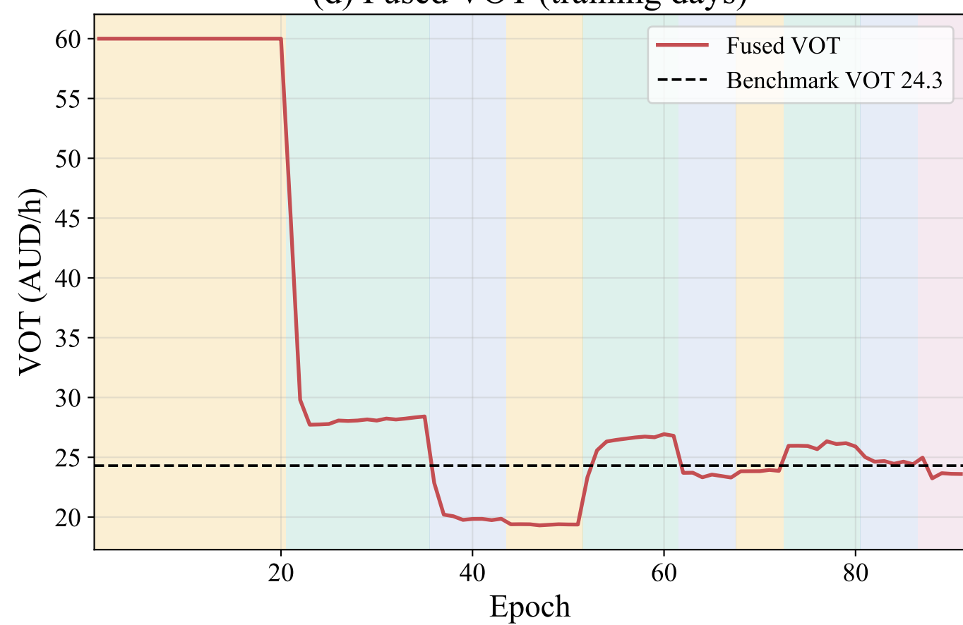
(d) Fused VOT (training days)
